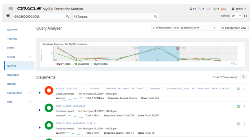
MySQL Query Analyzer 画面
